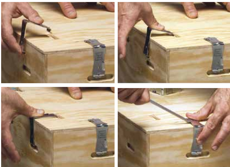
Montagesystem mit wiederverwendbaren Verriegelungslaschen
